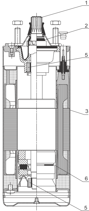
Fig. 17 MS 402 motor
