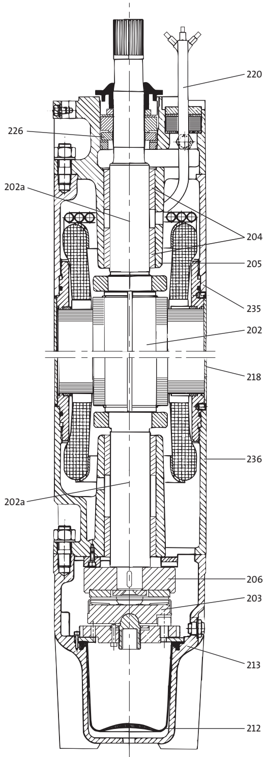
Fig. 20 MMS 10000
